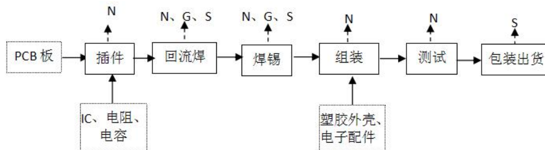
图 3-3 小夜灯生产工艺及产污环节流程图
