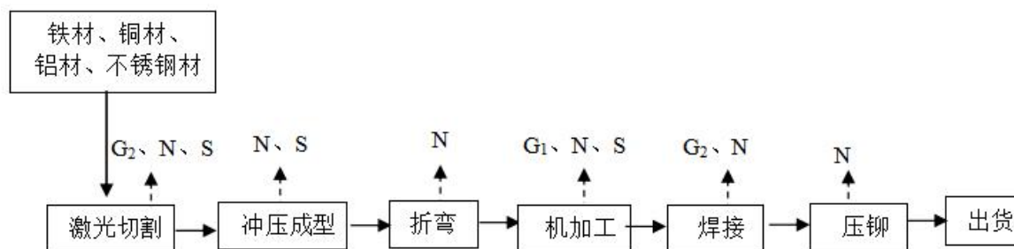
图 3-2 生产工艺及产污环节图
