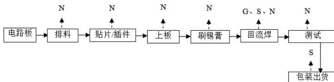
图 3-3 项目生产工艺及产污环节流程图
