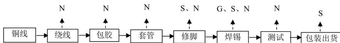
图 3-2 项目生产工艺流程及产污环节图
