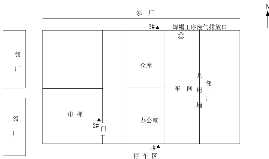
图 3-1 厂区平面布置及监测点位
